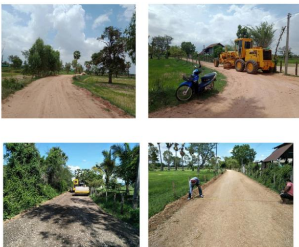
โครงการก่อสร้างถนนหินคลุก บ้านไร่อ้อย หมู่ที่ ๙ บริเวณเส้นทางจากหน้าวัดบ้านไร่อ้อยไปโคกหนองแวงบ้านหนองแจ้จ้อย (จ่ายขาดเงินสะสม)
