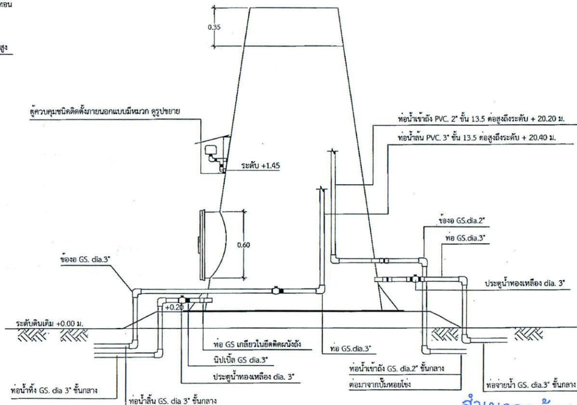
แบบแสดงการเดินท่อในถังแฉกเป๋ญ มาตราส่วน 1 : 25
