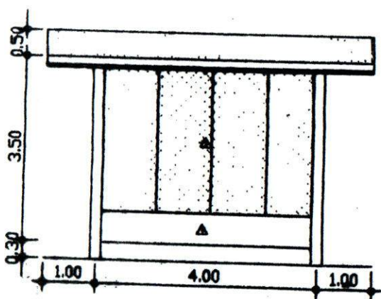
รูปด้านหลัง มาตรฐาน 1:100
