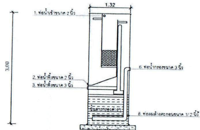
แบบแสดงส่วนประกอบภายในของถังกรอง
