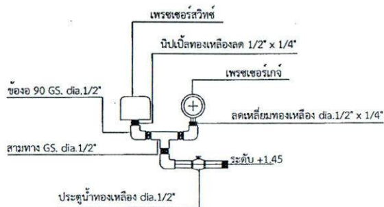
แบบขยายสวิตช์ควบคุมและแก้วัดความดัน
