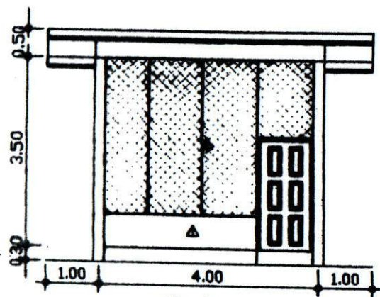
รูปด้านหน้า มาตรฐาน 1:100
