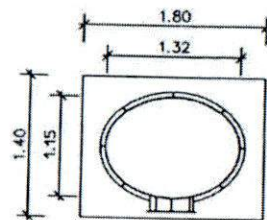
แบบแปลนถังกรองขนาด 20 ลบ.ม./ชม.
