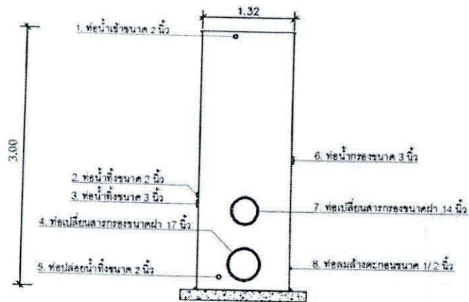
แบบแสดงส่วนประกอบภายนอกของถังกรอง
