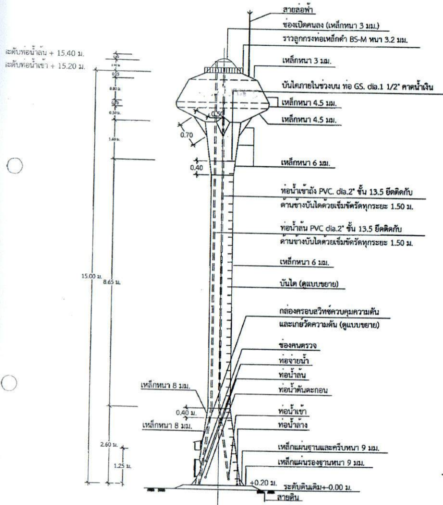
รูปด้านข้างท่อถึงสูง แบบถังเหล็กทรงถ้วยแชมเปญ
