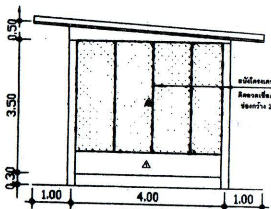
รูปด้านขวา มาตรฐาน 1:100
