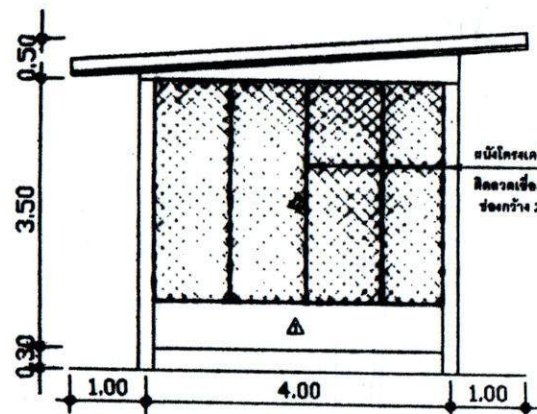
รูปด้านซ้าย มาตรฐาน 1:100
