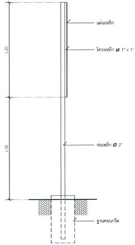
รูปด้านข้าง มาตรฐาน 1 : 20
